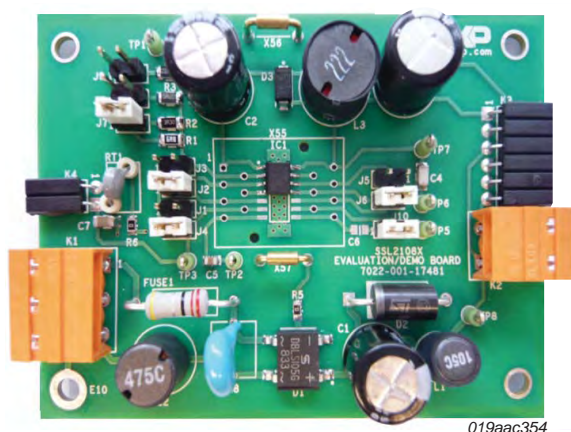
a. Top view: SSL21081 (SO8).
