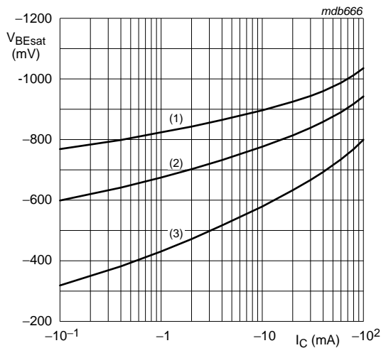
I_C/I_B = 10 (1) T_{amb} = -55 °C (2) T_{amb} = 25 °C (3) T_{amb} = 150 °C
