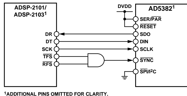
Figure 37. AD5382-to-ADSP-2101/ADSP-2103 Interface
