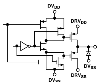
a) D0-D9
