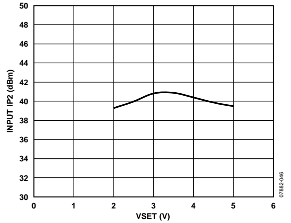
Figure 46. Input IP2 vs. VSET
