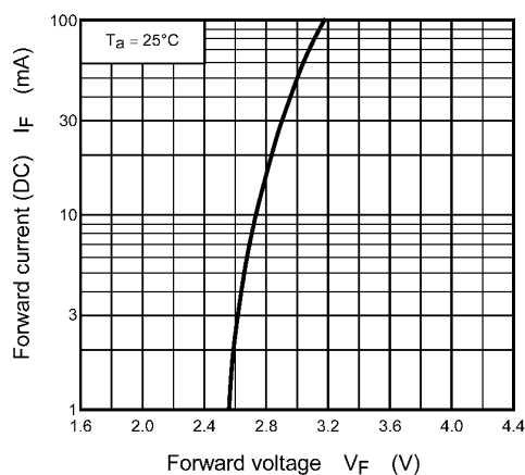
Fig. 8.1 I_F - V_F
