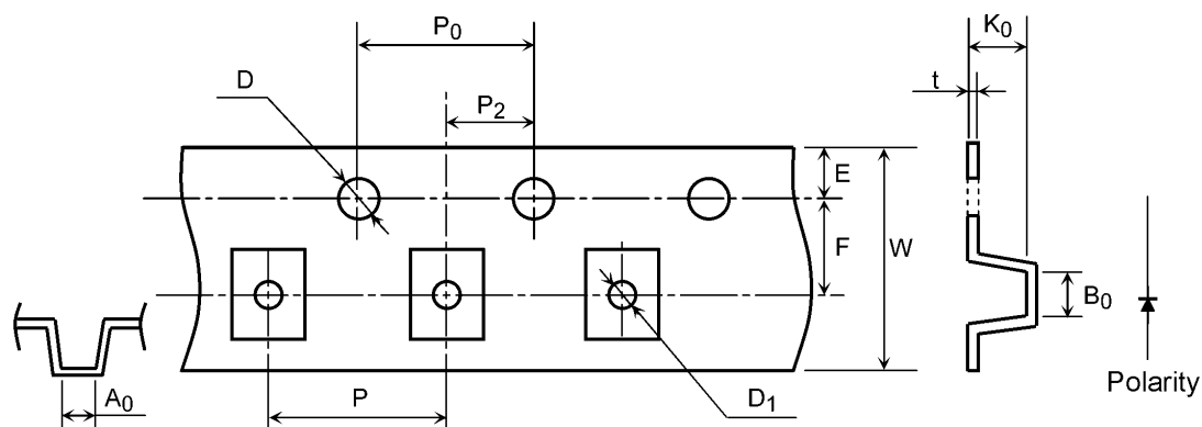
Fig. 12.3.1 Tape Dimensions
