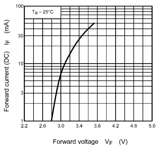
Fig. 8.1 I_F - V_F
