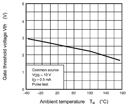
Fig. 8.9 V_{th} - T_a (Note 7)
