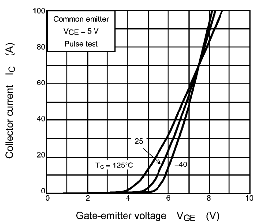
Fig. 8.5 I_C - V_{GE}
