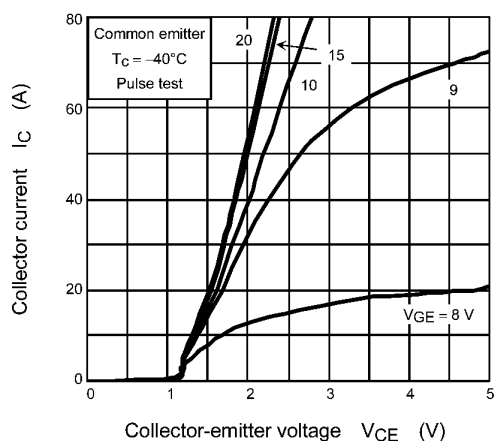
Fig. 8.1 I_C - V_{CE}
