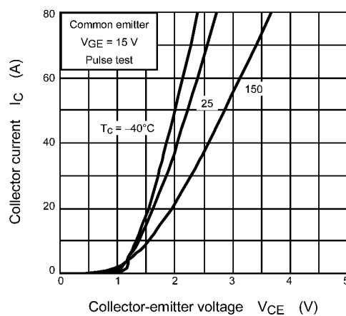
Fig. 8.4 I_C - V_{CE}
