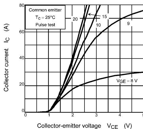
Fig. 8.2 I_C - V_{CE}
