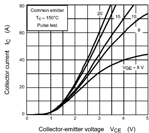
Fig. 8.3 I_C - V_{CE}
