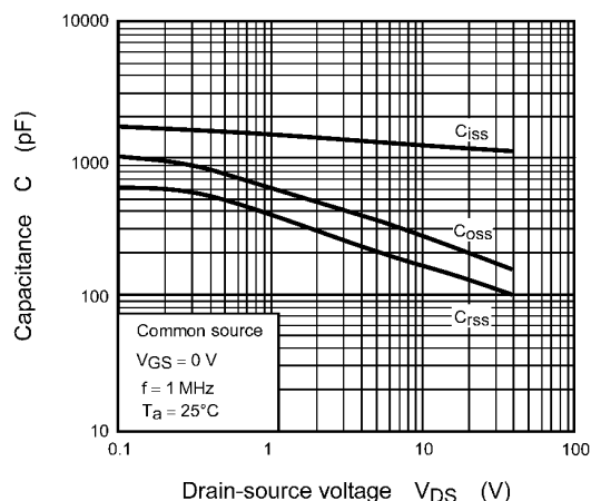
Fig. 8.8 Capacitance - V_{DS}
