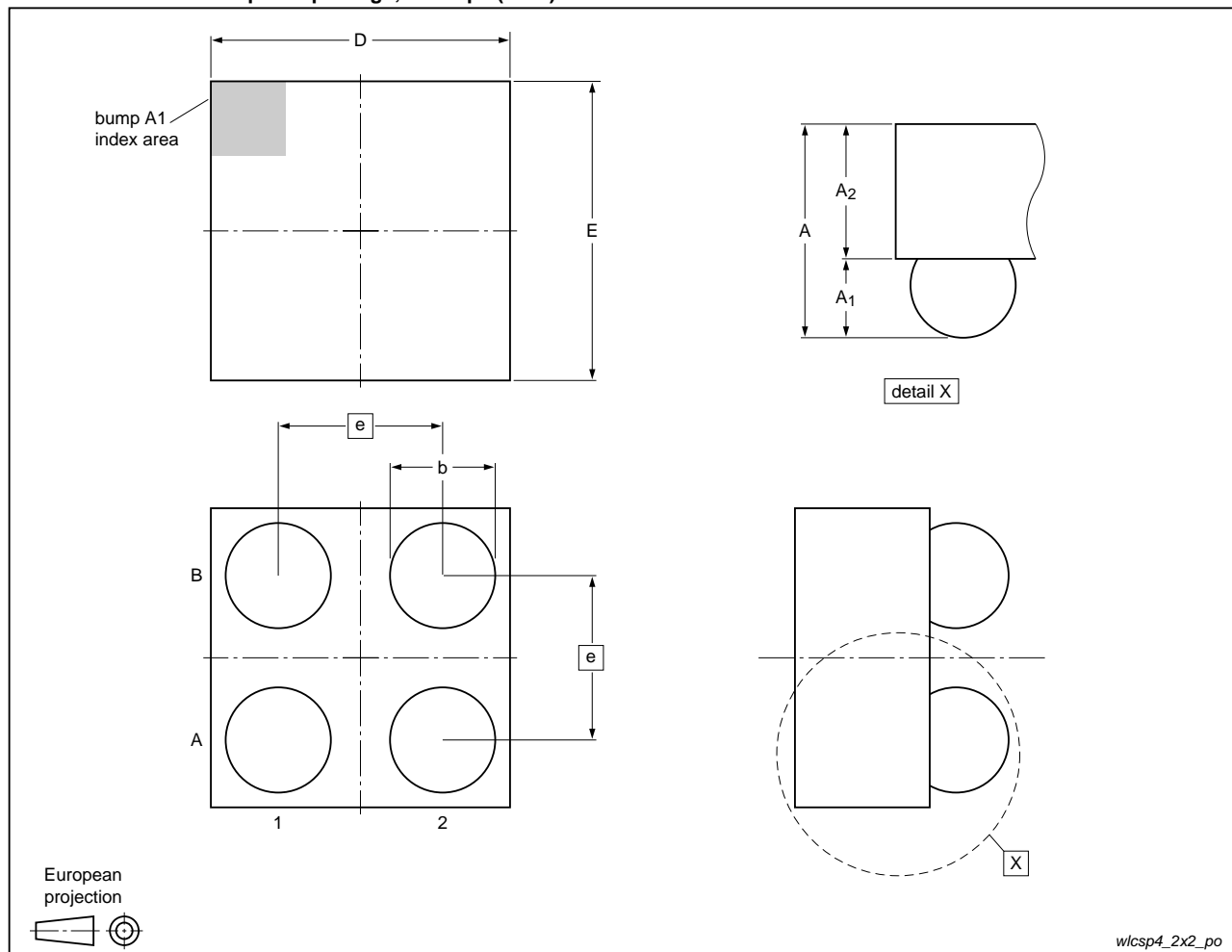
Fig 24. Package outline WLCSP4
