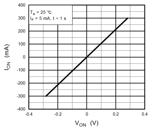
Fig. 12.1.4 I_{ON} - V_{ON}
