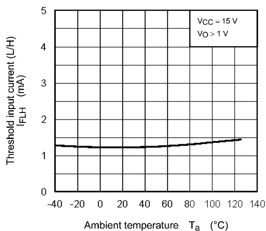
Fig. 12.2.4 I_{FLH} - T_a
