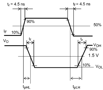
図 12.1.5 伝搬遅延時間測定回路, 波形
