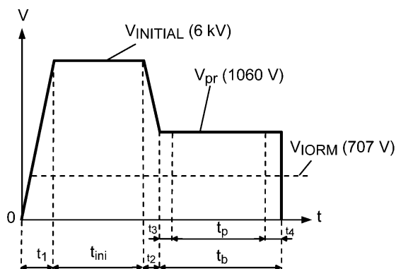
ダイアグラム 2 EN60747 による試験電圧波形、手順 b)、非破壊試験(全数試験に適用)
