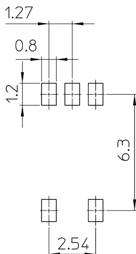
図 14.1 参考パッド寸法 (unit: mm)
