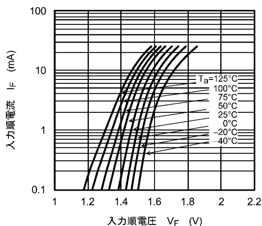
図 12.2.1 I_F - V_F
