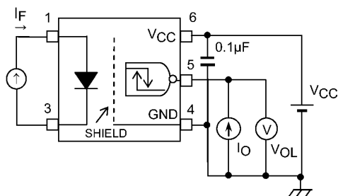
図 12.1.1 VOL測定回路
