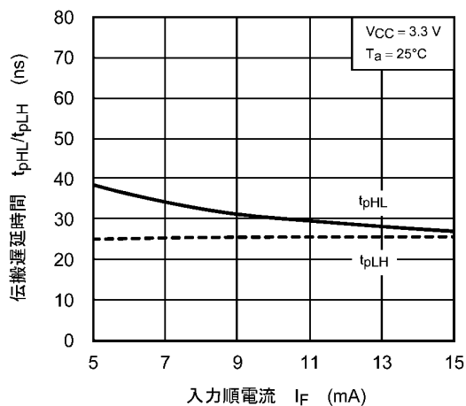
図 12.2.13 t_{pHL}/t_{pLH} - I_F
