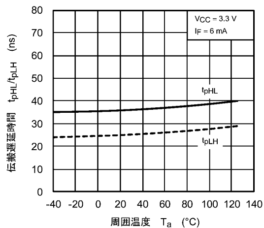
図 12.2.9 t_{pHL}/t_{pLH} - T_a
