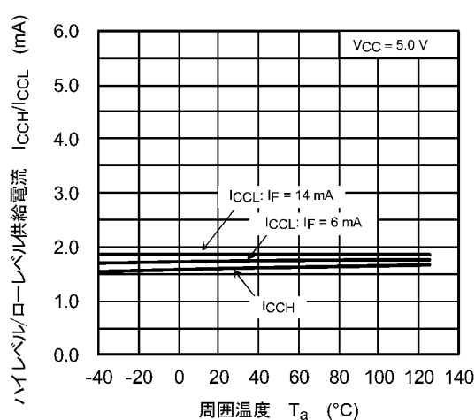
図 12.2.6 I_{CCH}/I_{CCL} - T_a
