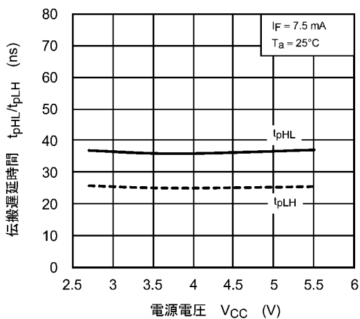
図 12.2.17 t_{pHL}/t_{pLH} - V_{CC}
