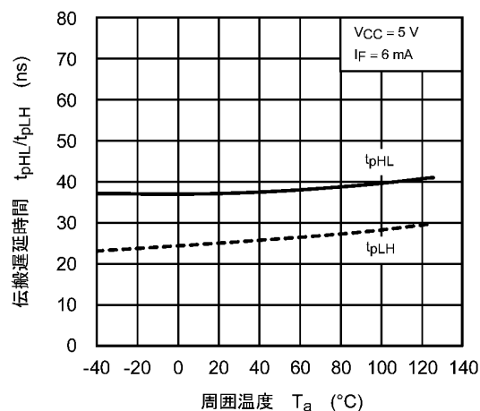
図 12.2.11 t_{pHL}/t_{pLH} - T_a
