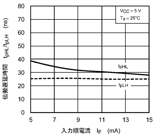
図 12.2.15 t_{pHL}/t_{pLH} - I_F
