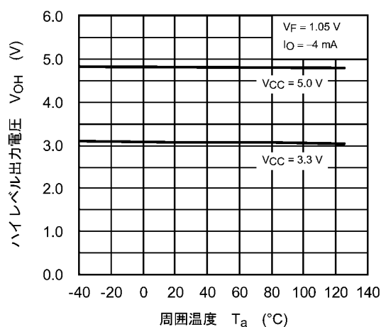
図 12.2.4 V_{OH} - T_a
