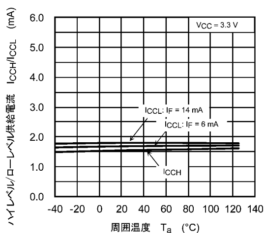
図 12.2.5 I_{CCH}/I_{CCL} - T_a
