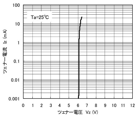
I_z - V_z
