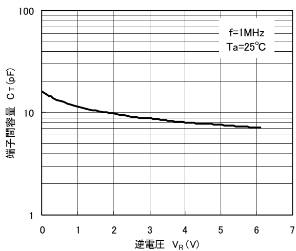
C_T - V_R
