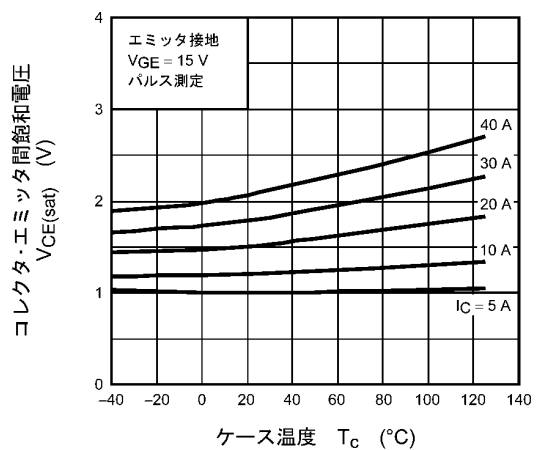
図 8.6 VCE(sat) - TC
