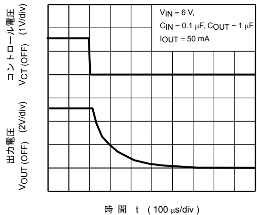
TCR5SB50U (出力立下り波形)
