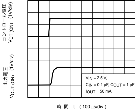
TCR5SB15U (出力立ち上がり波形)
