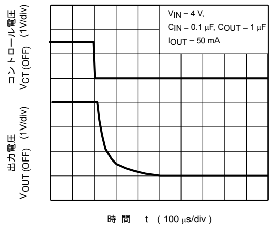
TCR5SB30U (出力立下り波形)
