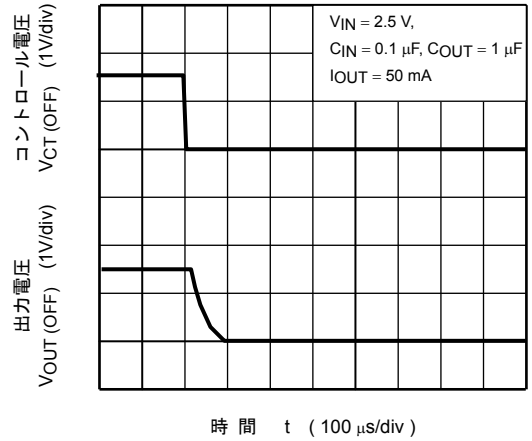
TCR5SB15U (出力立下り波形)
