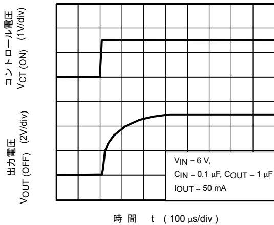
TCR5SB50U (出力立ち上がり波形)
