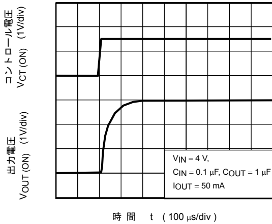
TCR5SB30U (出力立ち上がり波形)
