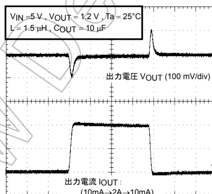
負荷応答特性
