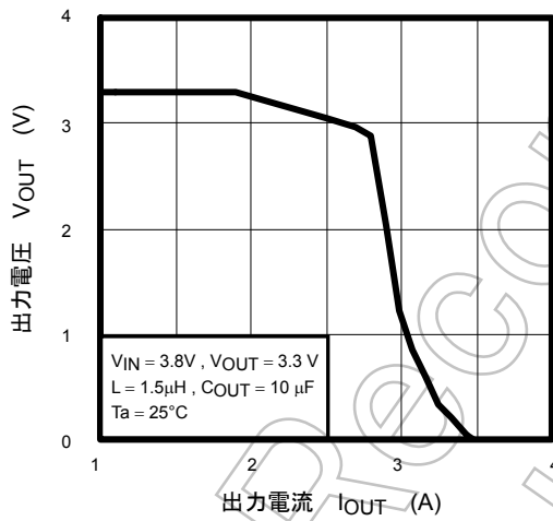
過電流特性
