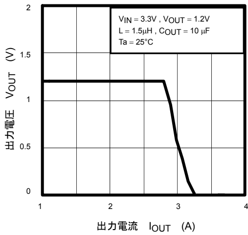
過電流特性
