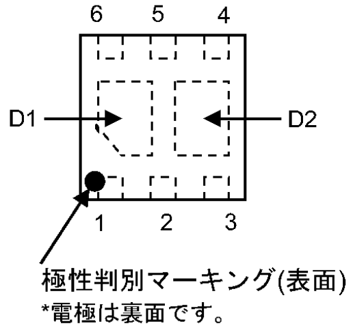
図 6.2 ピン配置(Top View)
