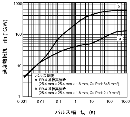
図 7.13 r_{th} - t_w
