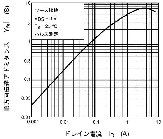
図 7.8 |Y_{fs}| - I_D
