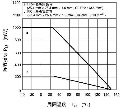
図 7.14 P_D - T_a
