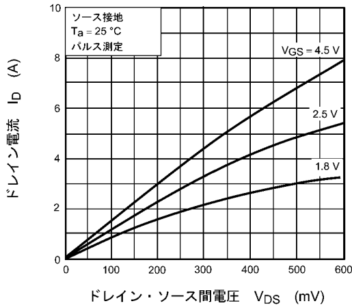
図 7.1 I_D - V_{DS}
