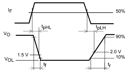
図 12.1.6 伝搬遅延時間測定回路, 波形
