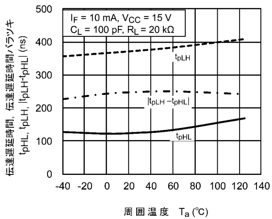
図 12.2.10 t_{pHL}, t_{pLH}, |t_{pLH} - t_{pHL}| - T_a
