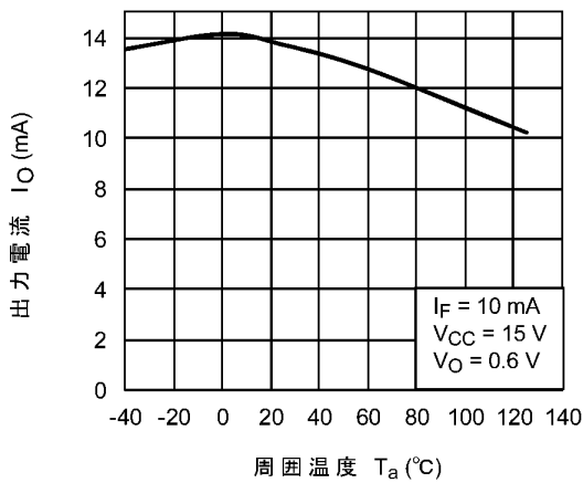
図 12.2.5 I_O - T_a
