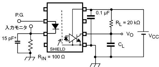
図 12.1.6 伝搬遅延時間測定回路, 波形
