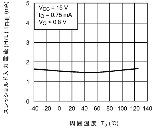
図 12.2.2 I_{FHL} - T_a
