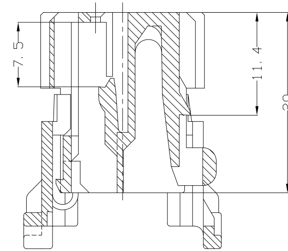
SECTION A-A (SCALE: 2.5/1)
