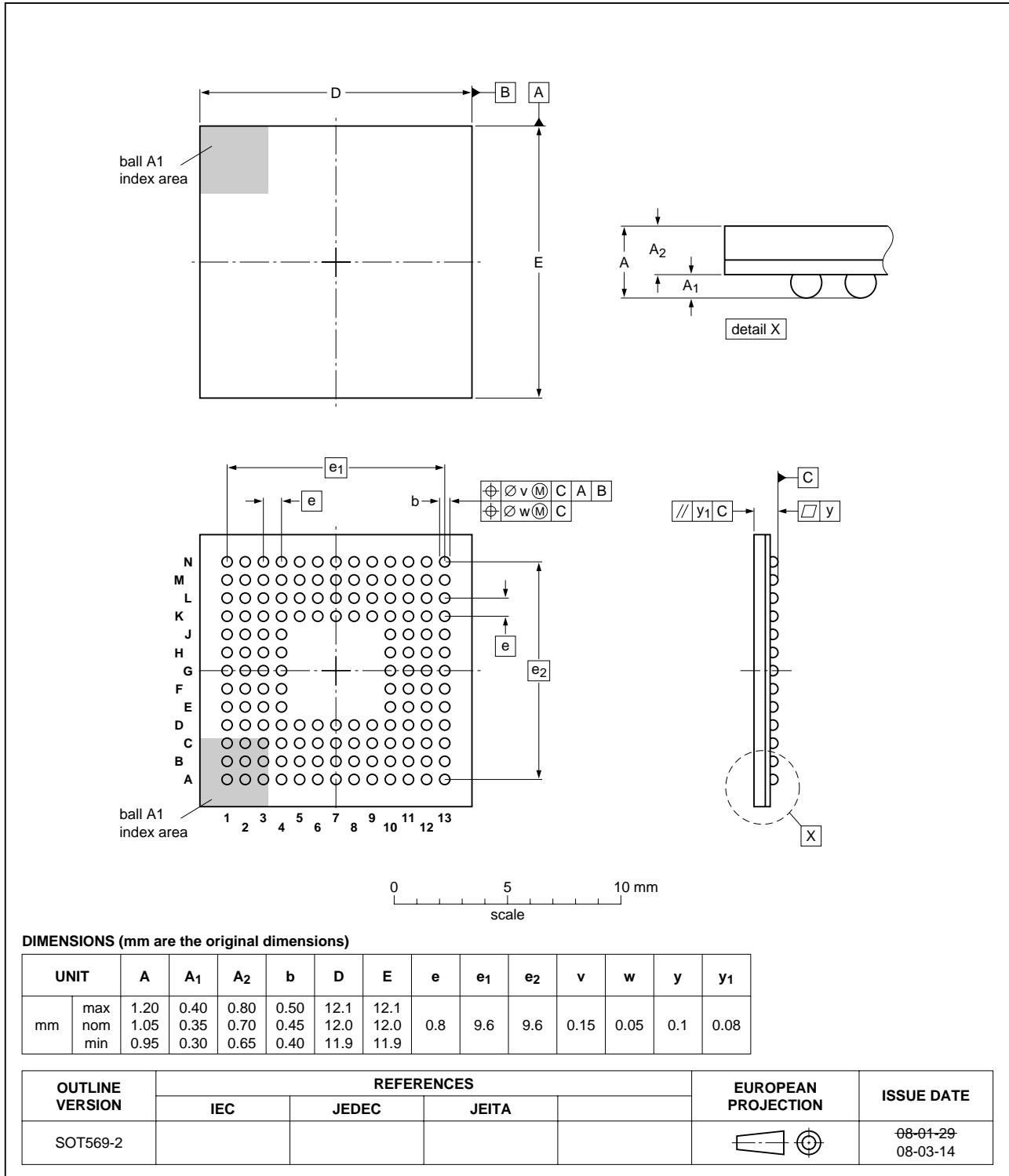
SOT569-2
