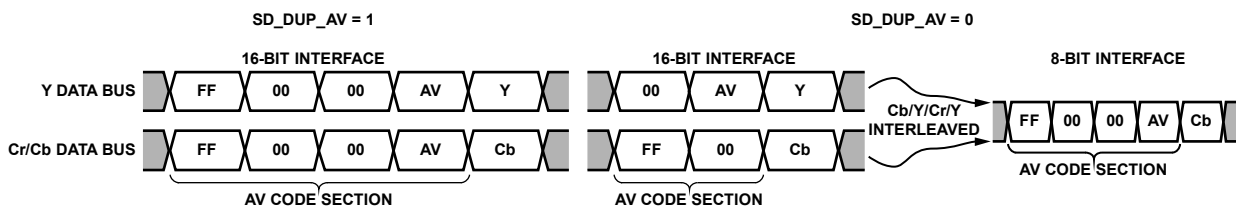
Figure 30. AV Code Duplication Control (64-Lead LQFP Only)
