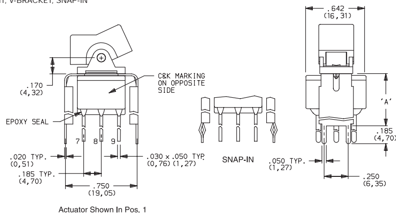
E301J1_BE2 3PDT
