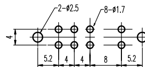
基板孔参考图 (指定外公差±0.05)
