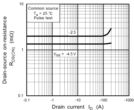
Fig. 8.5 R_{DS(ON)} - I_D
