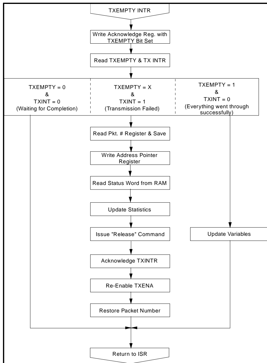
Figure 8.4 -TXEMPTY INTR
