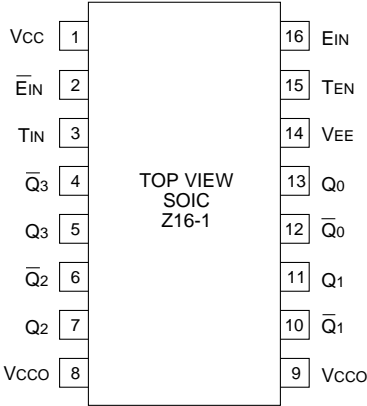
16-Pin SOIC (Z16-1)
