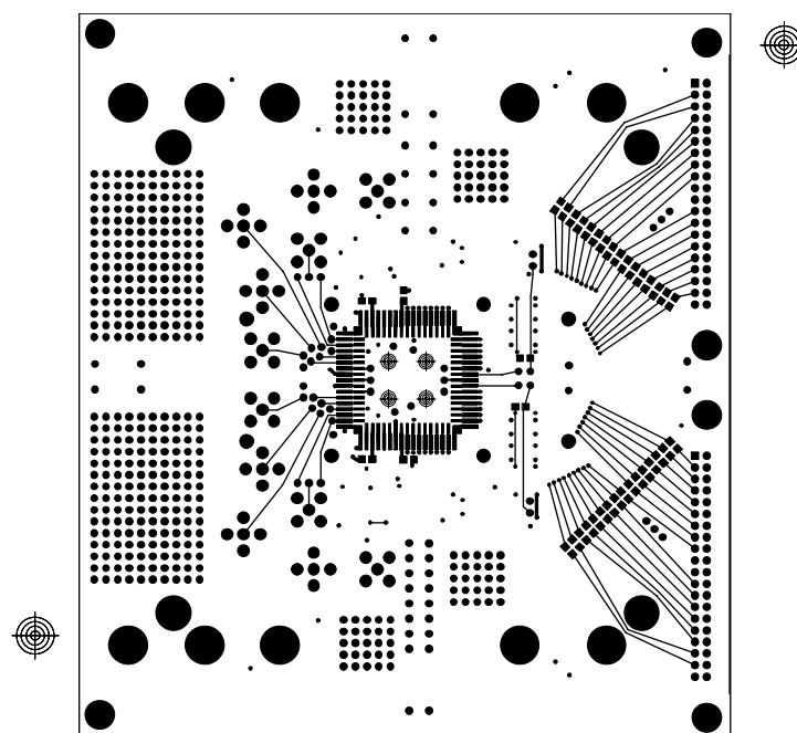
Figure 25. Top Layer
