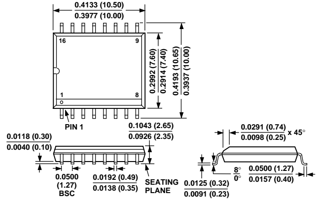
SOIC (R-16)
