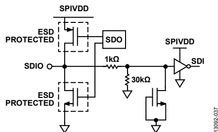
Figure 37. SDIO Input
