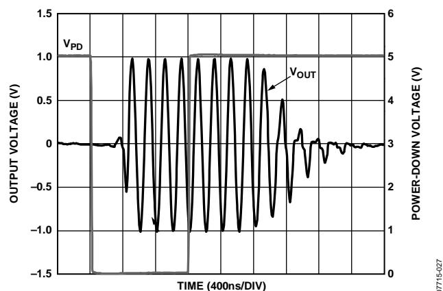
Figure 27. Enable/Power-Down Time
