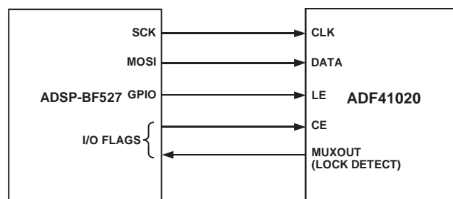
Figure 19. ADSP-BF527-to-ADF41020 Interface
