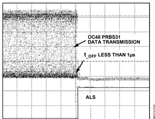
Figure 13. ALS Assert Time, 5 μs/DIV
