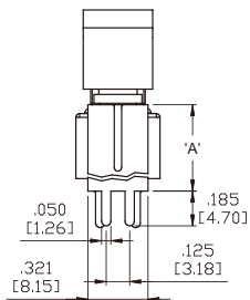
VS2-VS3 Double Pole
