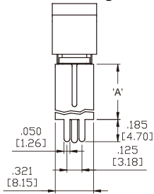
VS2-VS3 Single Pole
