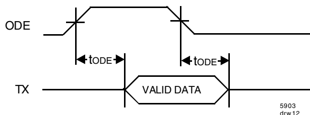
Figure 10. Output Driver Enable (ODE)
