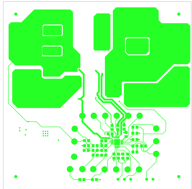
FIGURE 24. TOP LAYER
