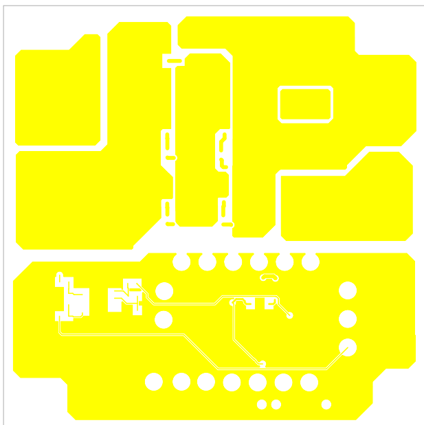
FIGURE 27. BOTTOM LAYER
