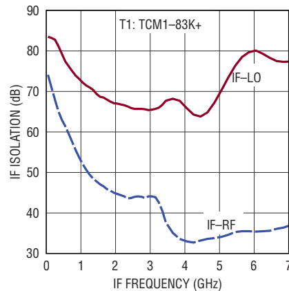
IF Isolation
