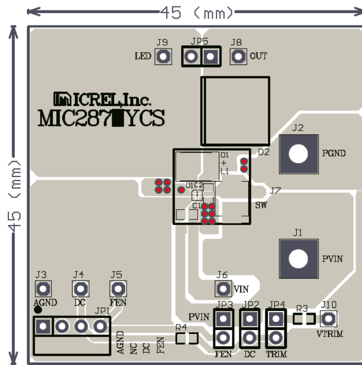
Top Layer
