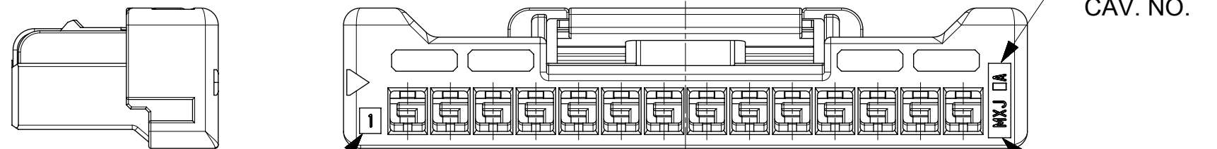
8-15CKT.外觀形状 8-15CKT. APPEARANCE FORM
