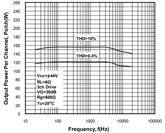
Po-f STK433-330N-E
