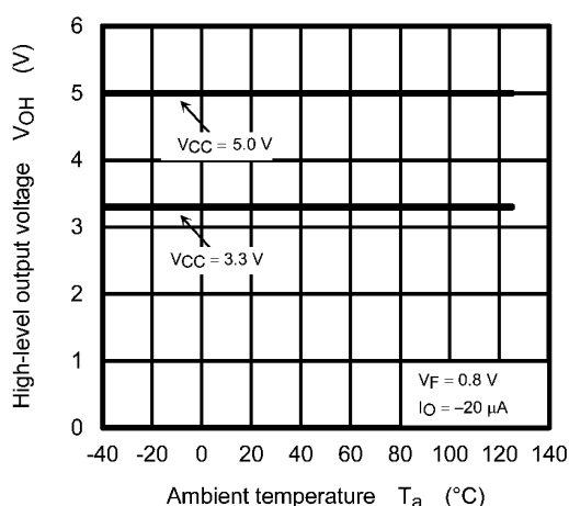
Fig. 12.2.5 V_{OH} - T_a
