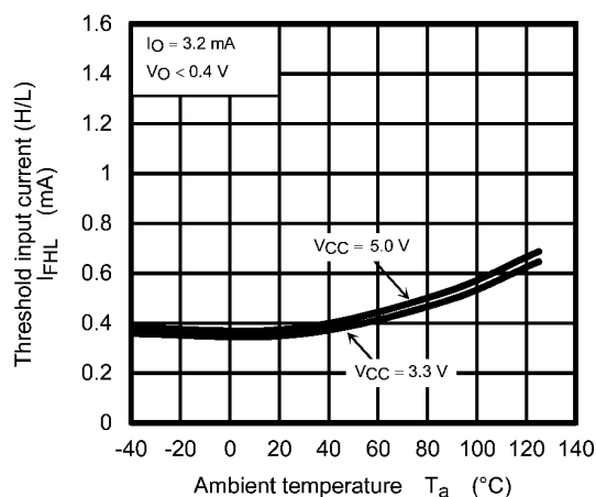
Fig. 12.2.9 I_{FHL} - T_a
