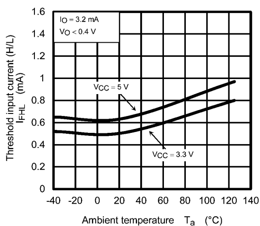
Fig. 12.2.9 I_{FHL} - T_a
