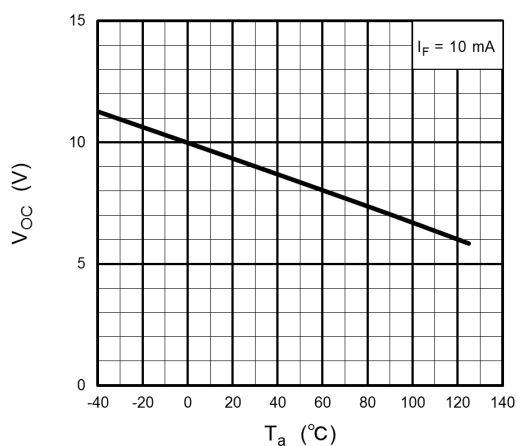
Fig. 12.5 V_{OC} - T_a
