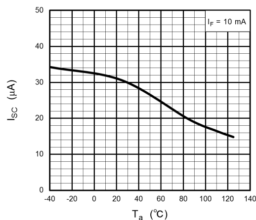
Fig. 12.6 I_{SC} - T_a
