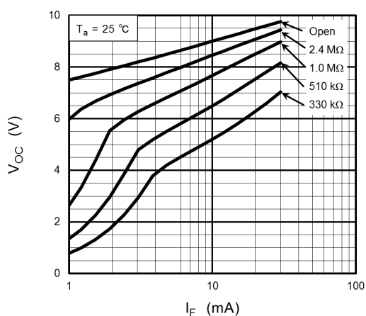
Fig. 12.3 V_{OC} - I_F
