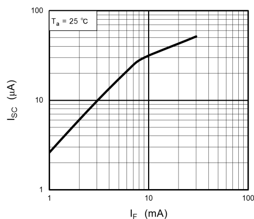
Fig. 12.4 I_{SC} - I_F
