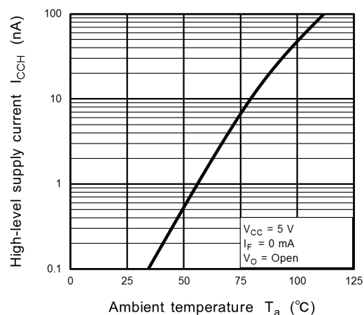
Fig. 12.2.4 I_{CCH} - T_a
