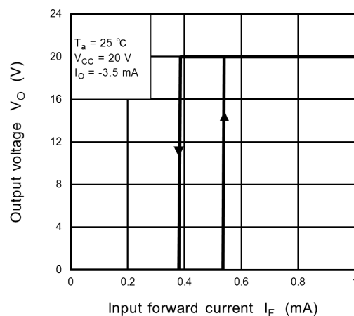
Fig. 12.2.4 V_O - I_F(I_{HYS})
