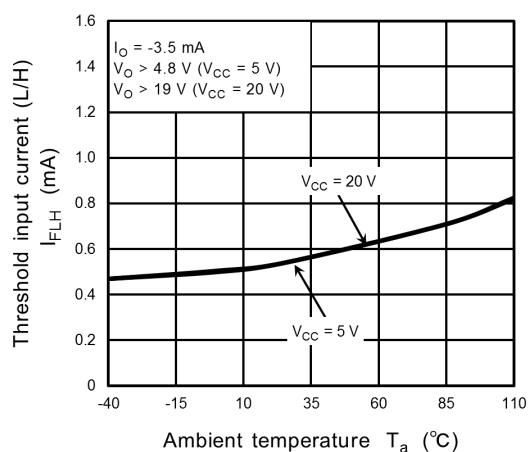
Fig. 12.2.2 I_{FLH} - T_a
