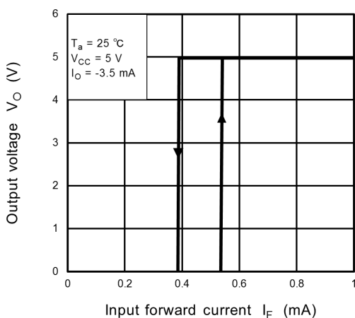
Fig. 12.2.3 V_O - I_F(I_{HYS})
