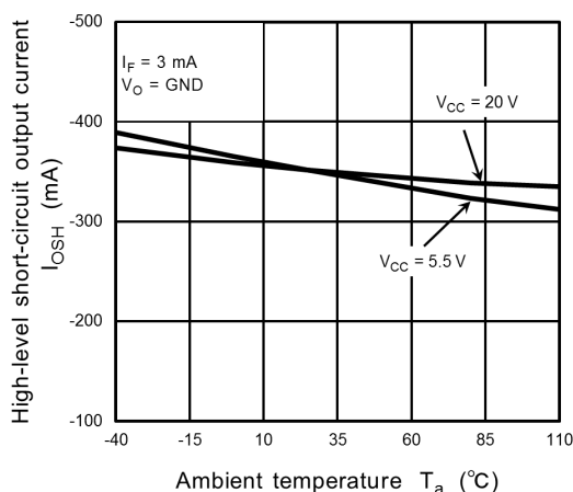
Fig. 12.2.10 I_{OH} - T_a
