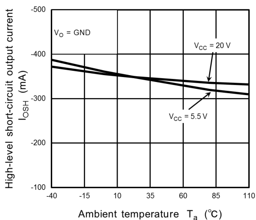
Fig. 12.2.10 I_{OH} - T_a
